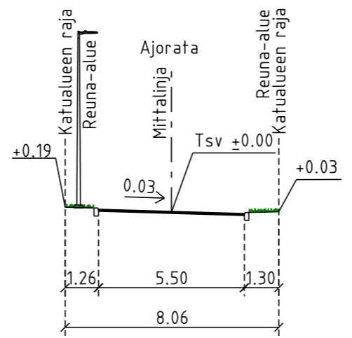
LEIKKAUS C-C 1:200
