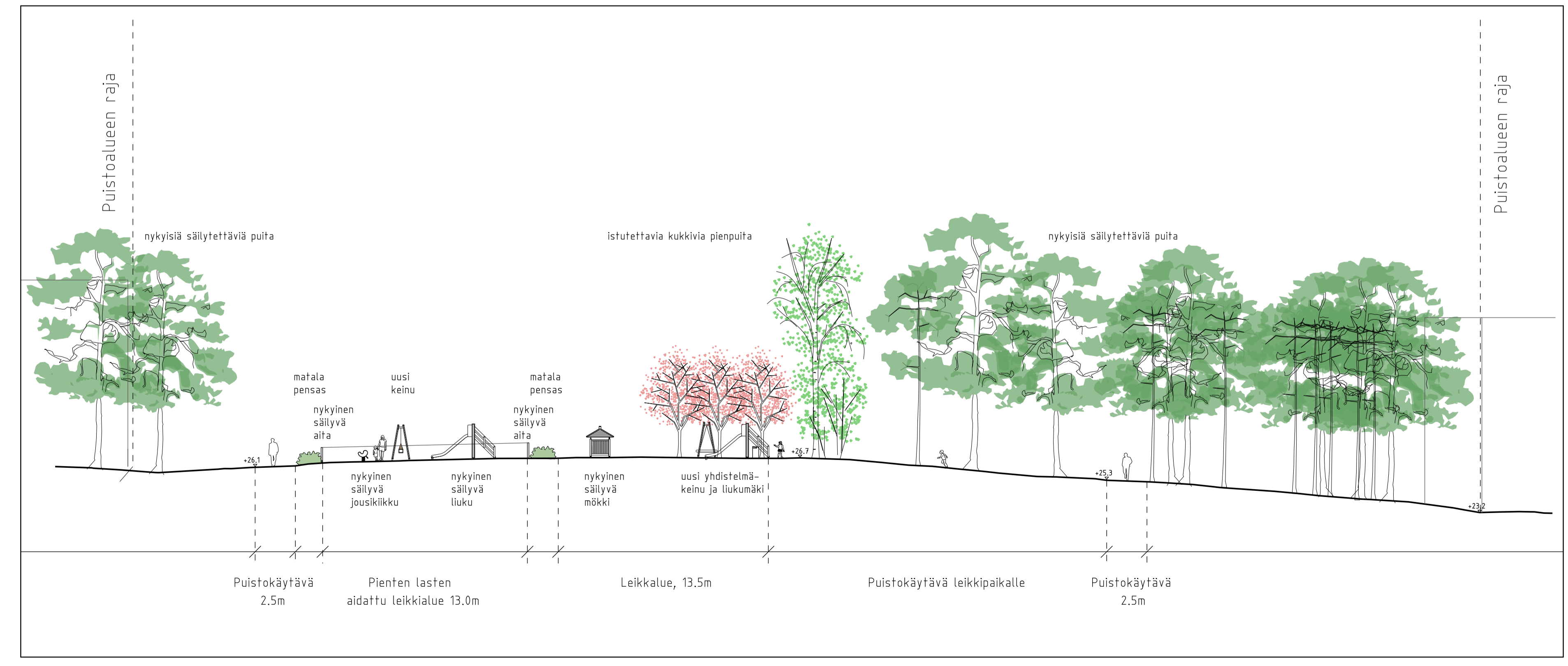
Tyyppiopikkileikkaus A-A, 1:200
