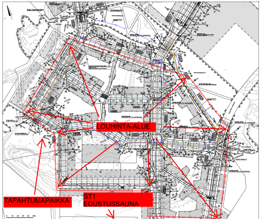
Kuva 1. Louhintakohde
