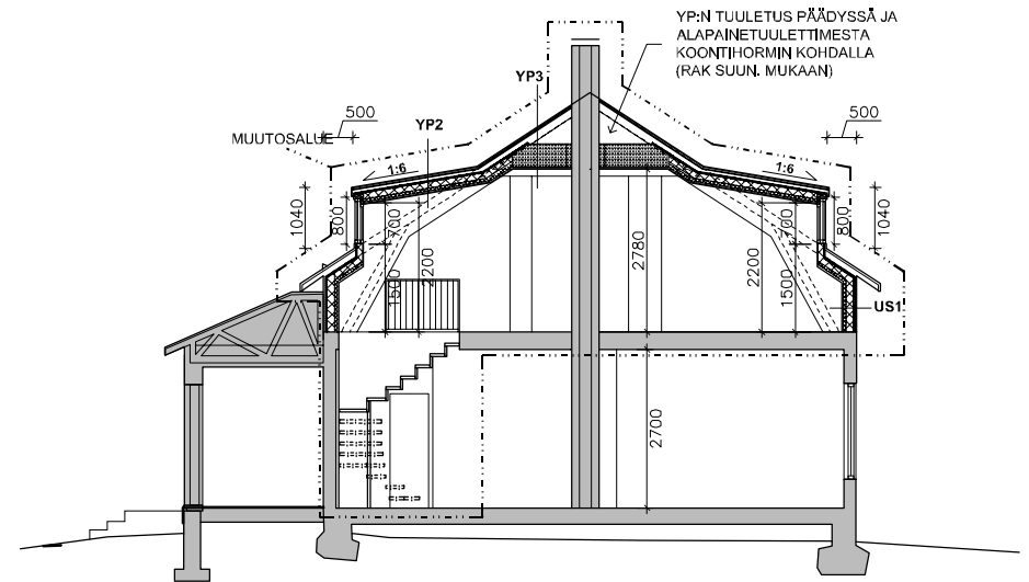
POIKKILEIKKAUS
