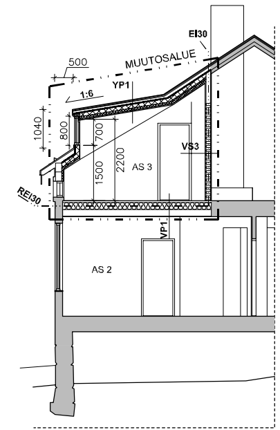
POIKKILEIKKAUS
