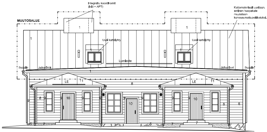
JULKISIVU LUOTEeseen
