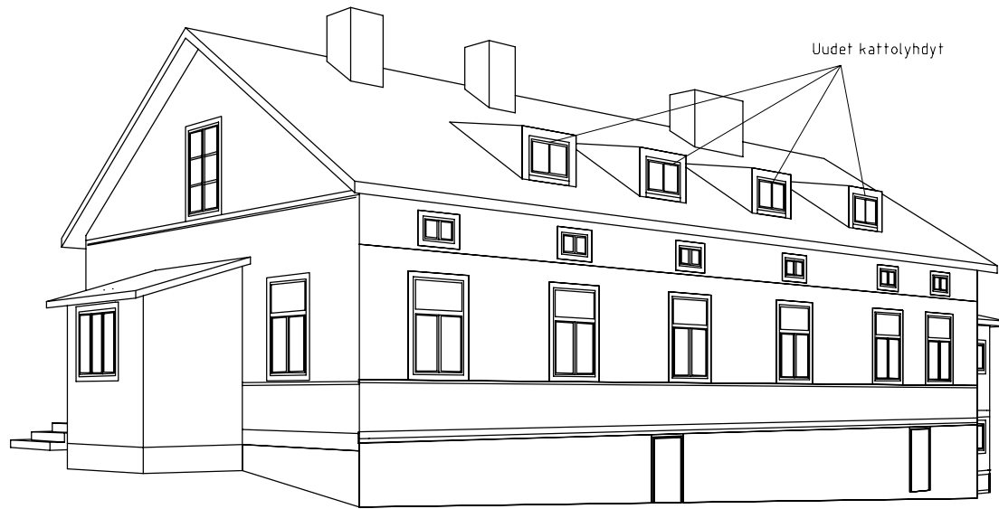
KATTOLYHDYT, MASSOITTELU TAKAJULKISIVU, RAK 2
