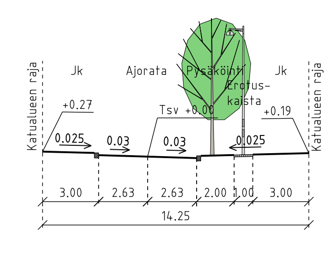
Kultaveneenkatu M-M
