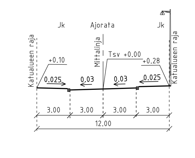
Kultakruunuankaari K-K
