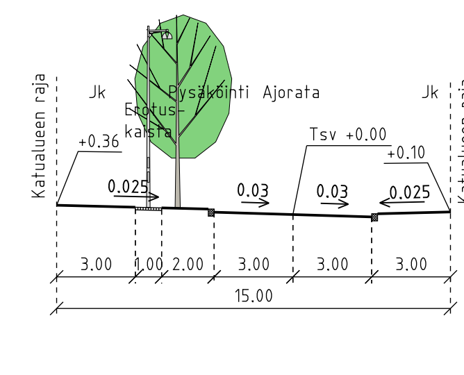
Kultaveneenkatu L-L
