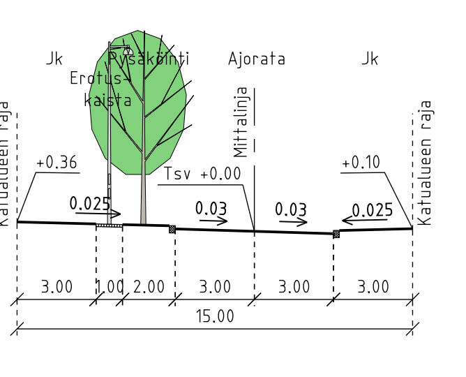
Kultakruunuankaari J-J
