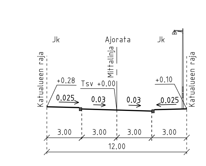
Kultakruunuankaari H-H
