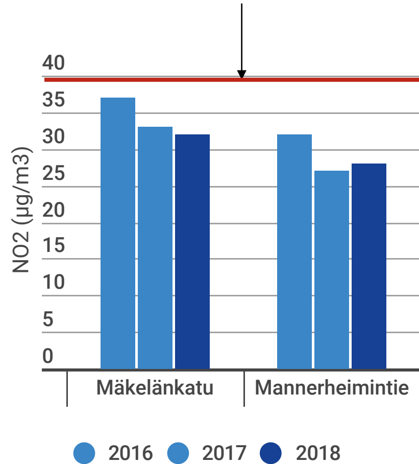
Tavoite NO2 ei ylitä 40 µg/m3 (EU-direktiivi 2024)
