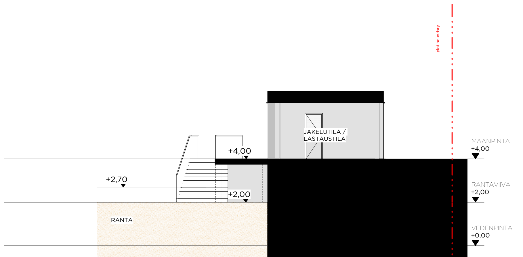
LEIKKAUS B-B
